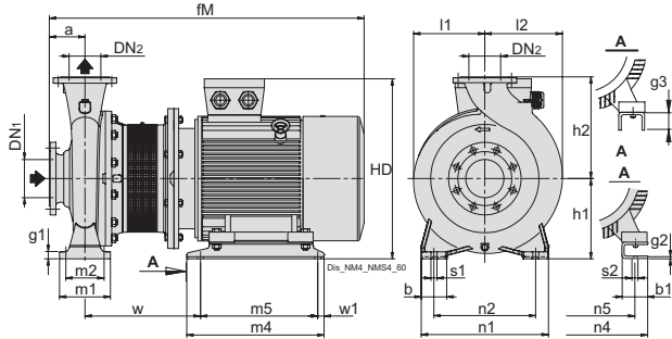
Brides EN 1092-2
