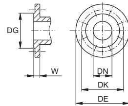
Brides EN 1092-2
