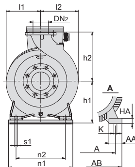
Brides EN 1092-2
