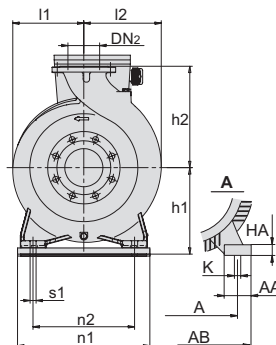
Brides EN 1092-2
