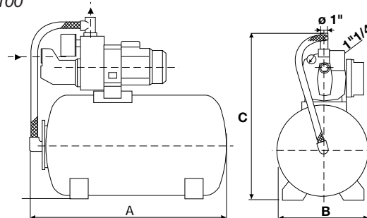
AQUAJET GWS 151/100
