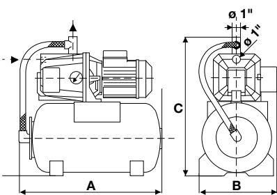
AQUAJET GWS 112/60 - 102/-60 - 132/100
